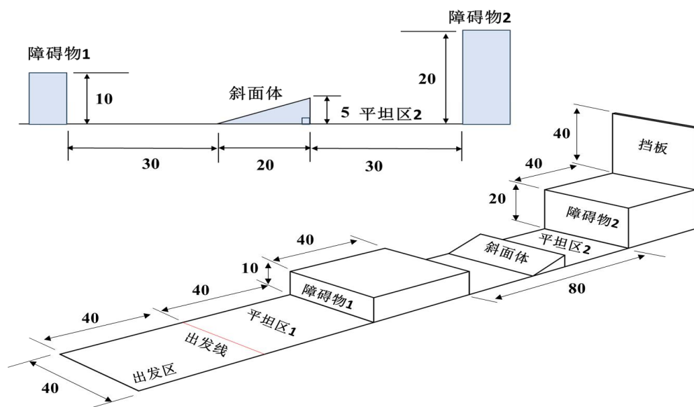
图4 复赛赛道立体及局部示意图
